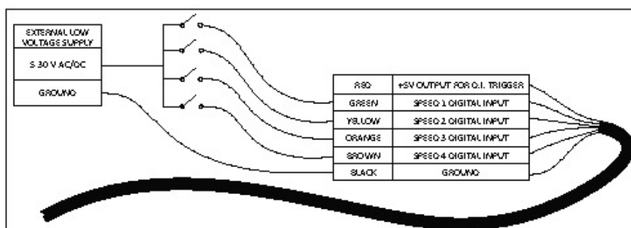
Figure 5 : Schéma de câblage d'alimentation électrique basse tension
