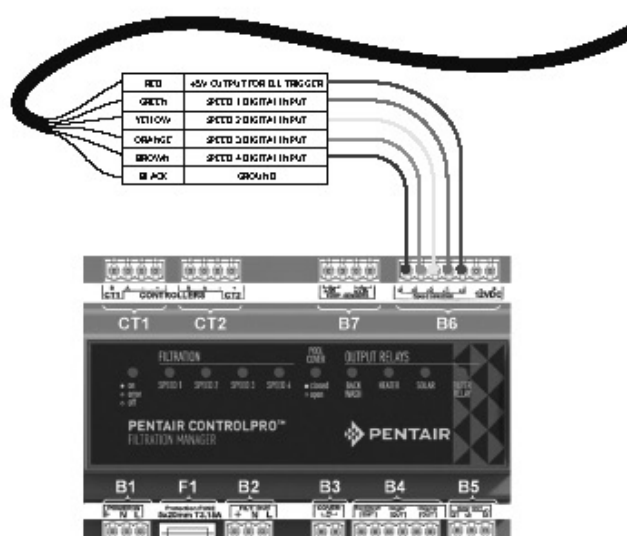
Figure 6 : Schéma de câblage ControlPro+
