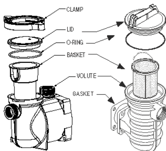
Ensemble de panier de pré-filtre
