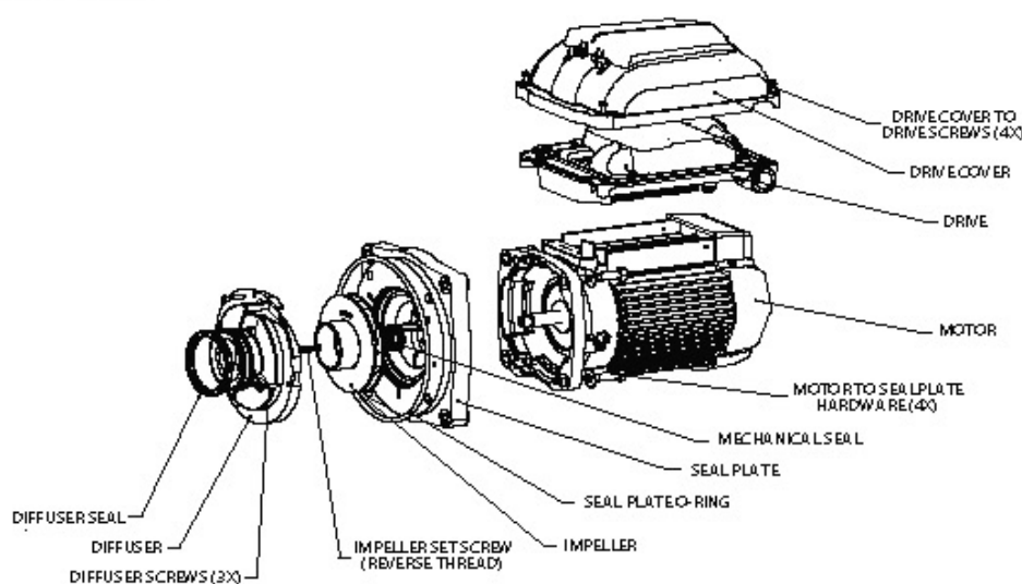
Assemblage du moteur SuperMax® VS2
